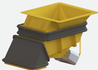
Podajnik wibracyjny
